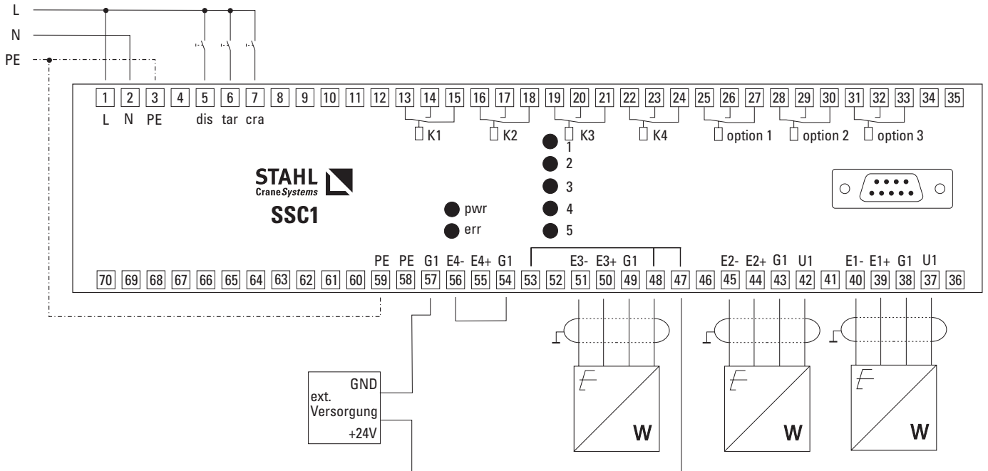
Relaiszuordnung Modus 1-2-3
